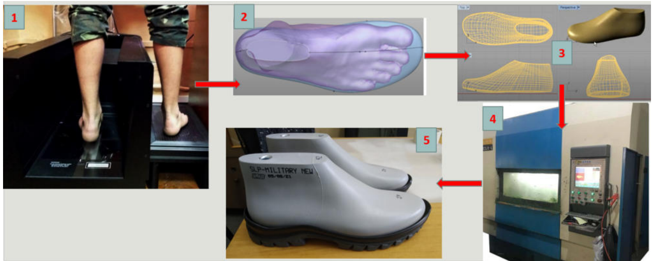
Рис. 3. Послідовність процесу розробки колодки на основі результатів 3д сканування
