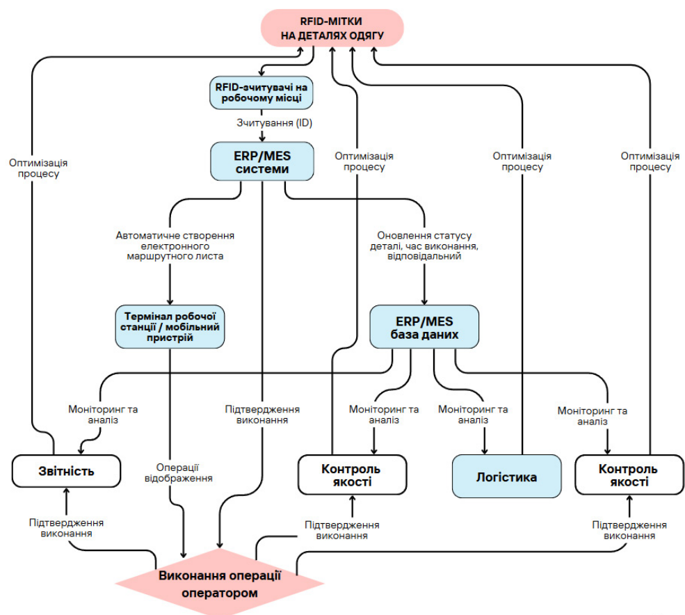
Рис. 1. Схема інтеграції RFID-технологій у виробничі процеси fashion-індустрії
