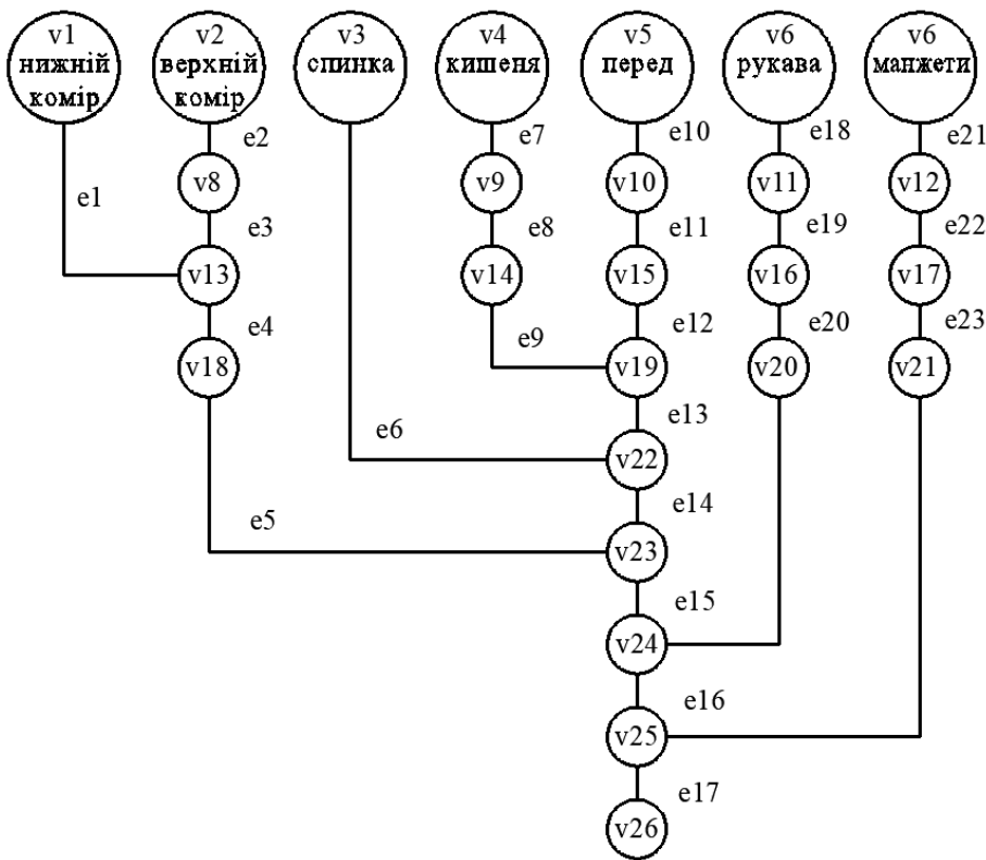
Рис. 2. Граф технологічного процесу виготовлення швейного виробу
